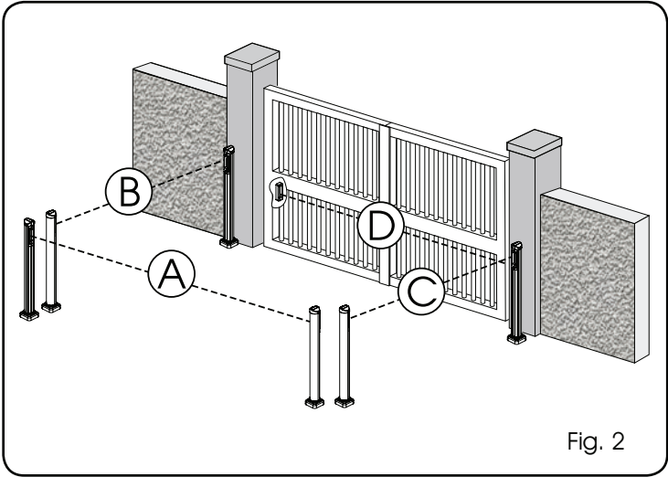
La fig. 2 illustre un automatisme pour portail battant à 2 vantaux avec les faisceaux de couverture des photocellules:
