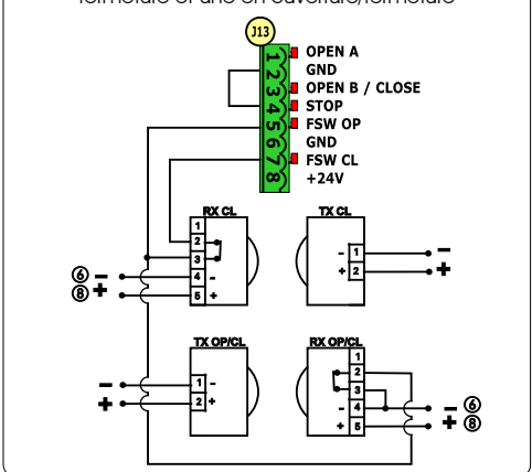
Branchement d'une paire de photocellules en fermeture, l'une en ouverture et l'autre en ouverture/fermeture
